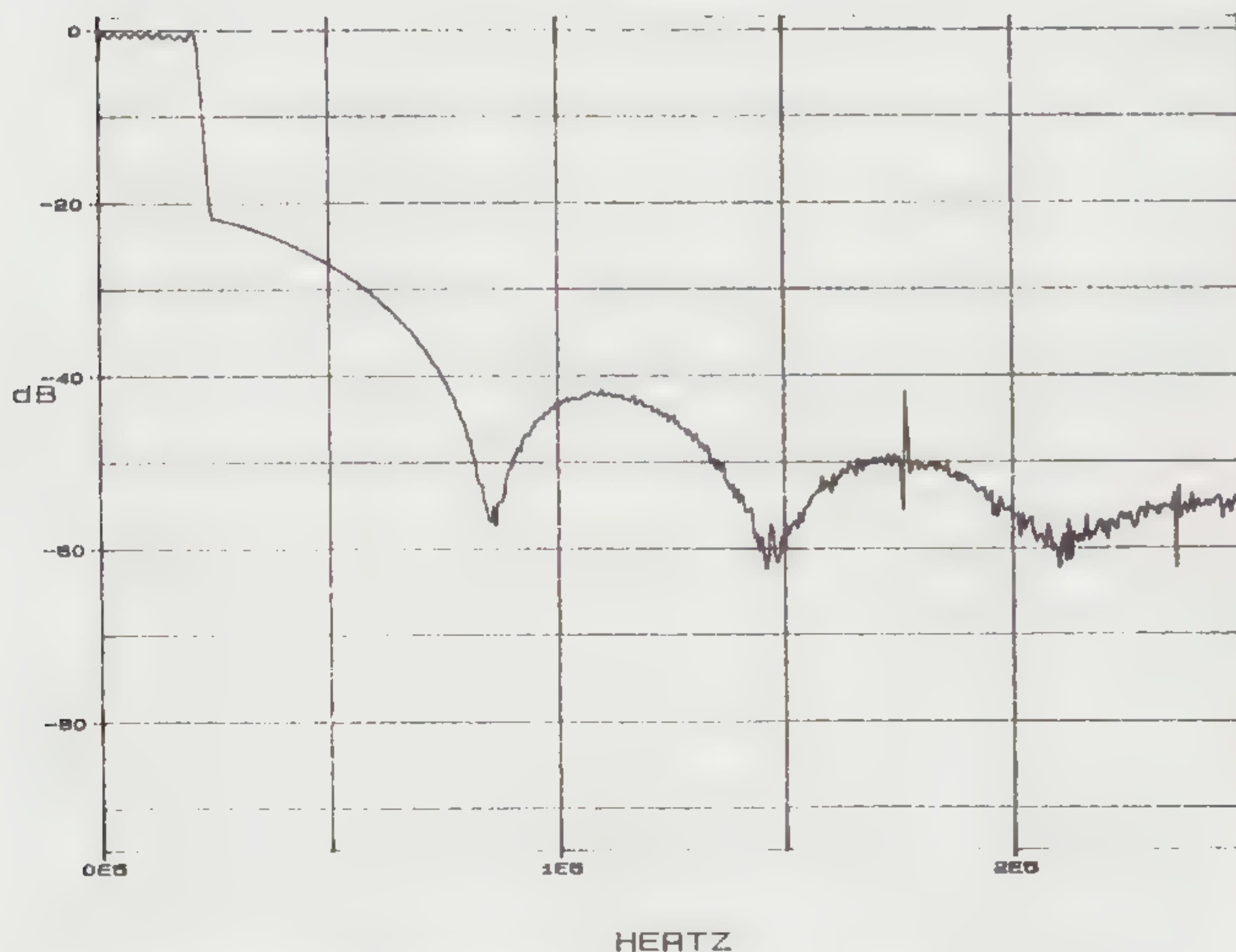
Figuur 6. Dc combinatie CD-A70 + AX-300. Tape Out
